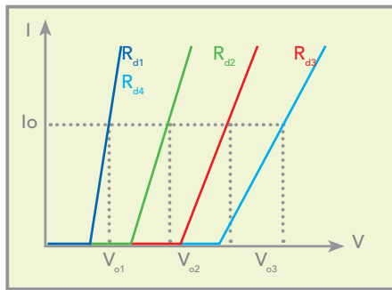
图 2 - 不同颗数LED模拟
